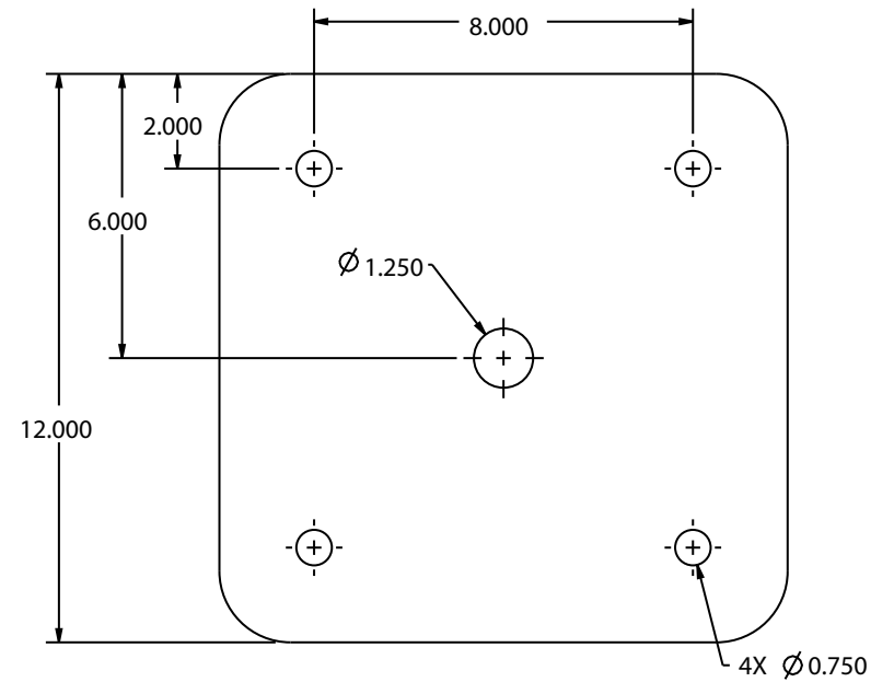
Bottom Baseplate
