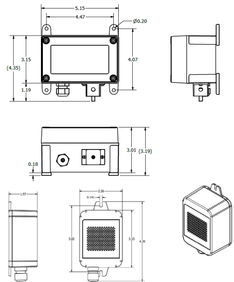
99122 - Optional Remote CO2
