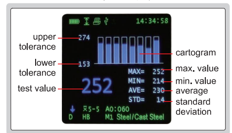
histogram display
